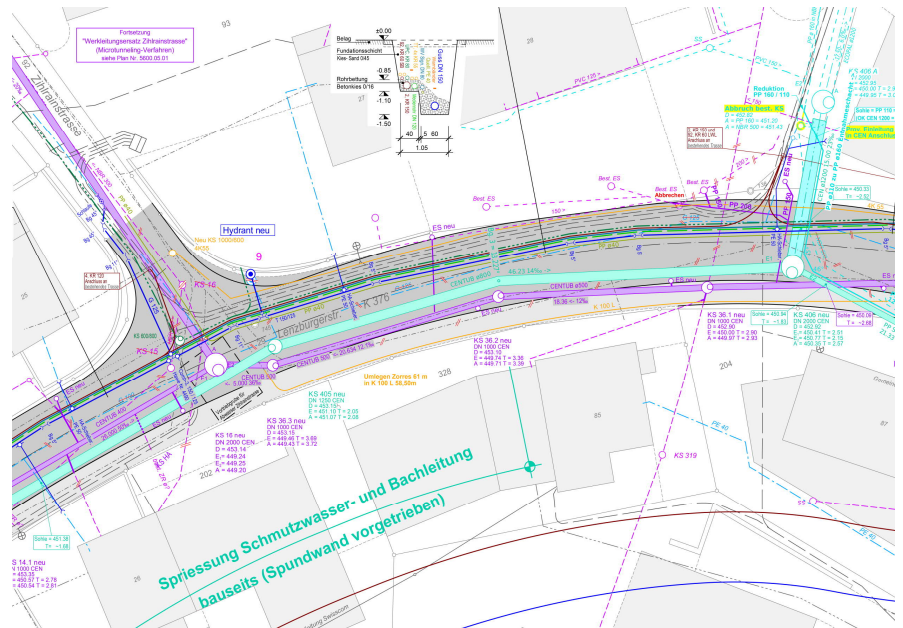
Kordinationsplan Kanalisation, Bachleitung, Wasserleitung, AEW, diverse Werke
