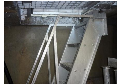
Neuer Eingang in Pumpensumpf über Ex-Geschützte Schachtabdeckung mit Steiltreppenkonstruktion
